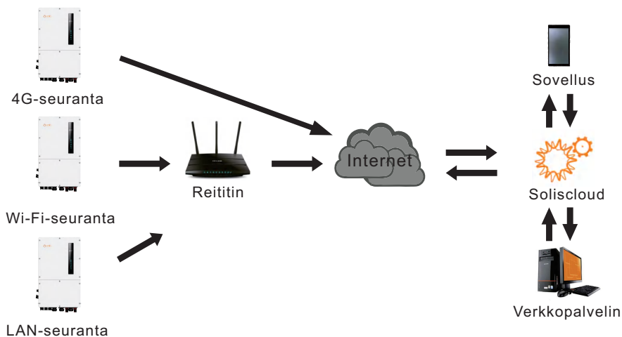
Kuva 3.33 Langaton tietoliikennetoiminto
