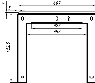
Kuva 3.6 Invertterin seinäasennus
