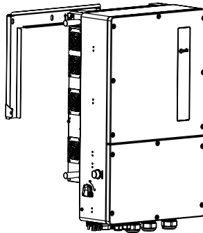
Kuva 3.7 Seinäkiinnike
