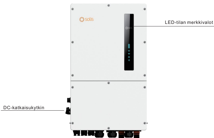
Kuva 1.1 Näkymä edestä
