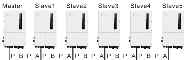
Kuva 3.22 Rinnakkaisliitäntä
